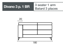
Materasso/Mattress/ Matelas 140 X 195 X h14 cm
